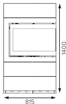
HWAM 5650
